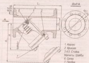
Конструкция фильтра ФСМ исп. 2
