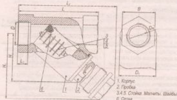
Конструкция фильтра ФСМ исп. 1
