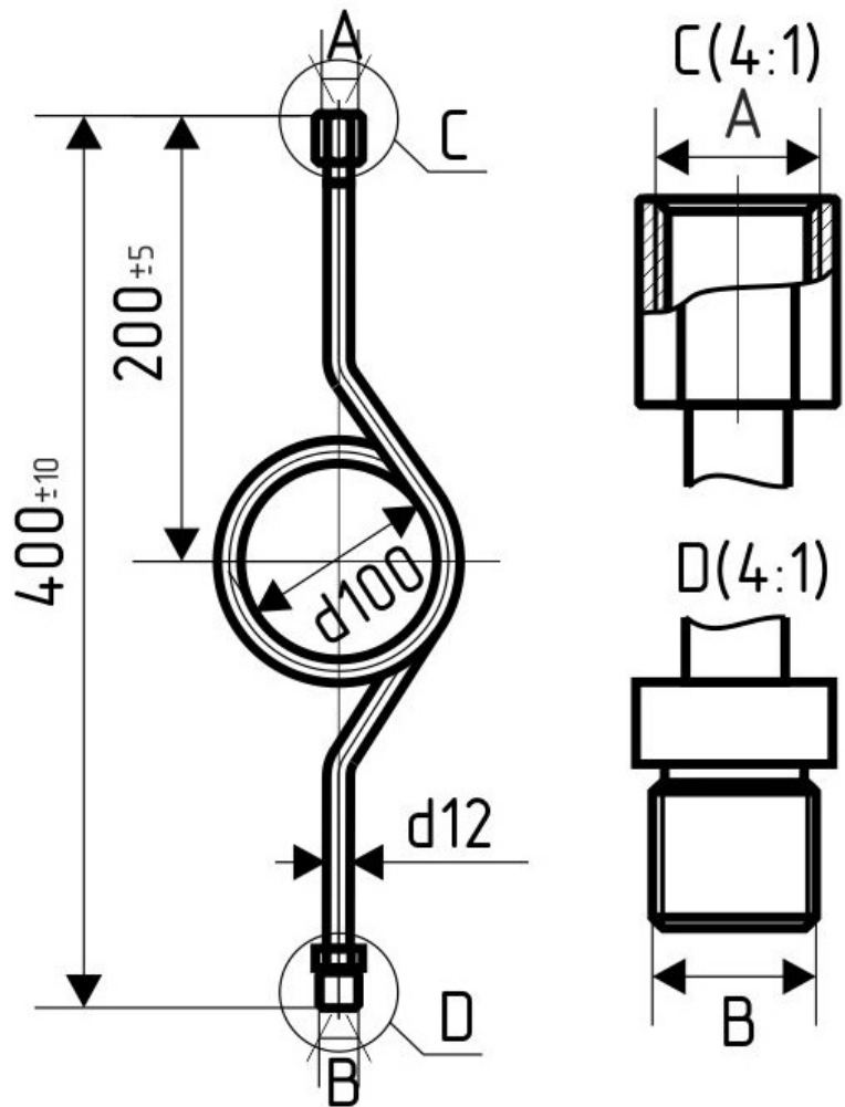
Отвод Оф100в-1
