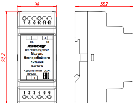
Приложение 1 Габаритный чертеж
