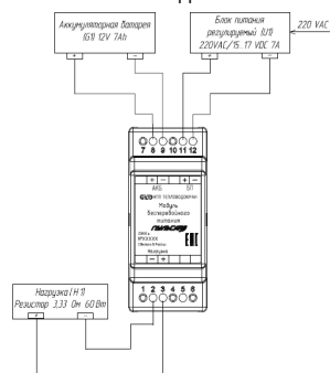
Приложение 2 Схема подключений
